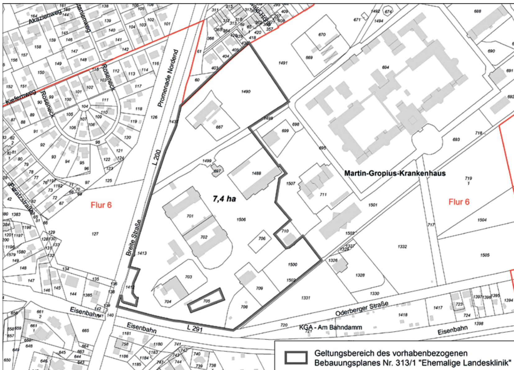
Vorhabenbezogener Bebauungsplan Nr. 313/1 „Ehemalige Landeslinik“
