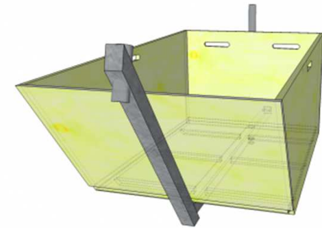
Entwurf der Transportkiste
