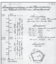
Leitungsplan um 1910, Eberswalde
